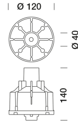
8945039 Controcassa Ø inner 40 / Ø outer 120 mm H. 160 mm
