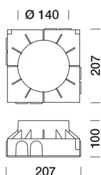
8945015 Controcassa Ø 140 mm H. 100 mm con base quadra 200 mm
