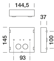
8945122 Controcassa per cartongesso/cemento TEAM Small
